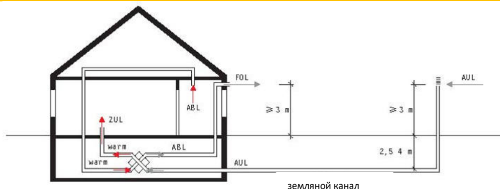
Рис. 5: Вентиляционная система с земляным каналом и рекуперацией тепла 20
