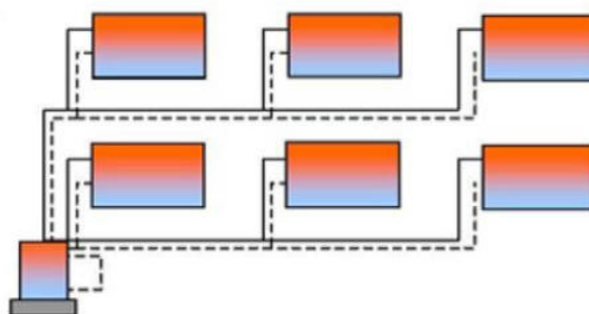
Рис. 12б: гидравлически сбалансированная система
