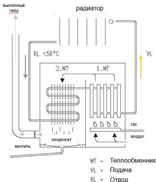
Рис. 7: Принцип конденсационного котла 5
