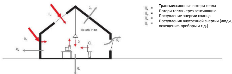
Рис. 4: Факторы, влияющие на тепловой баланс здания 2
